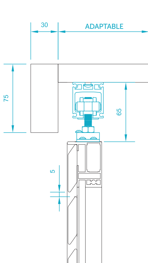
COULISSANT ALUMINIUM précadre alu 4 côtés pose sur façade avec ITE
