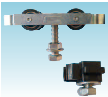
CHARIOT SUR ROULEMENT BUTEE FIN DE COURSE
