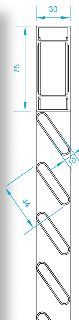
CADRE LAMES PERSIENNÉES à l'américaine
