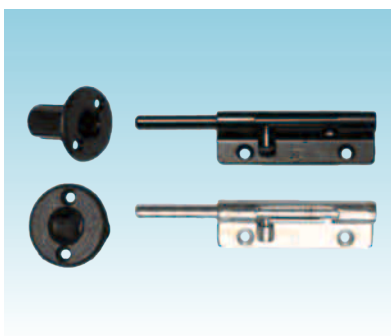
VERROU TARGETTE ALUMINIUM BRUT OU LAQUE RAL
