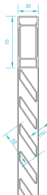
CADRE LAMES PERSIENNÉES à la française
